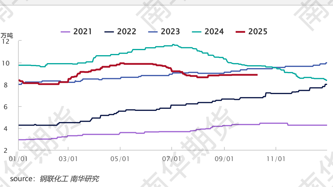
光伏玻璃日熔量季节性
