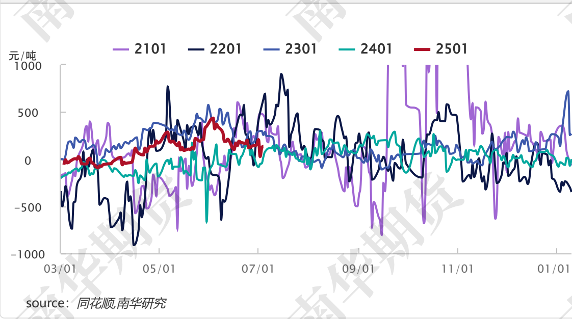
硅铁01合约基差季节性（宁夏）
