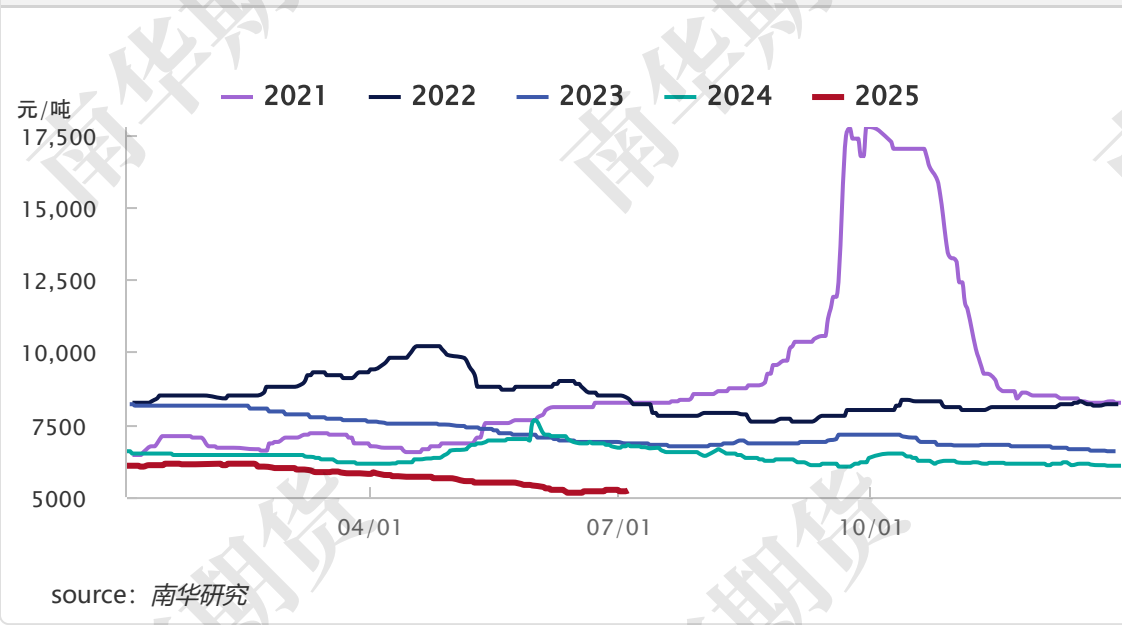
硅铁市场价季节性（内蒙 72%FeSi）
