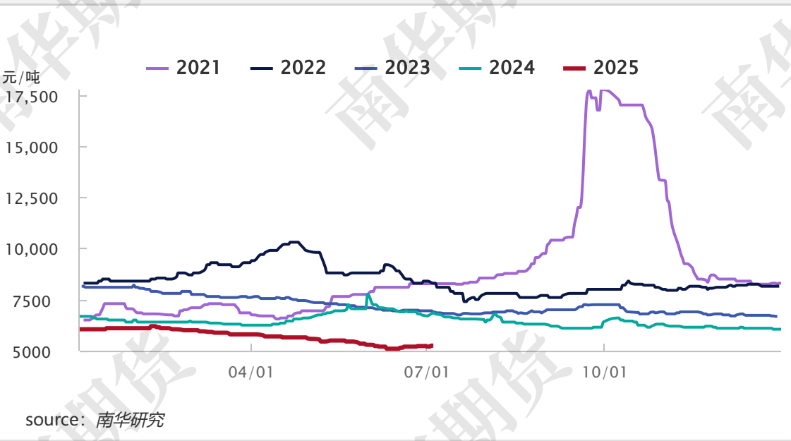
硅铁市场价季节性（宁夏 72%FeSi）
