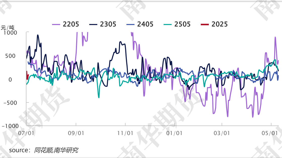
硅铁05合约基差季节性（宁夏）
